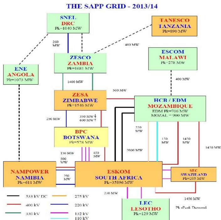
南部非洲国家间电网互联互通示意图
